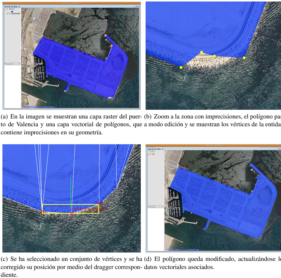
Figura 11: Ejemplo de edición de un polígono en gvSIG con la librería osgVP.
