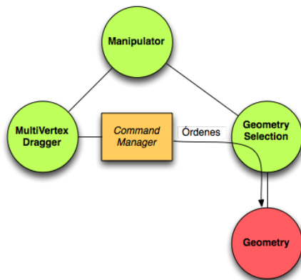
Figura 7: Grafo generado al crear un nodo GeometryManipulator . Se puede apreciar cómo las órdenes recibidas por el GeometrySelection son aplicadas directamente sobre la geometría.
