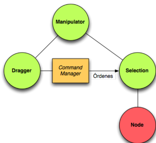
Figura 4: Arquitectura del nodo Manipulator. En él podemos observar los elementos que lo forman: Dragger, Selection y CommandManager.
