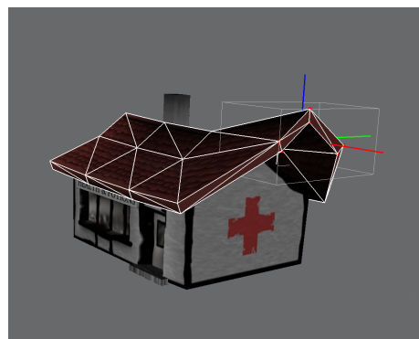
Figura 6: Nodo GeometryManipulator. Podemos observar los 3 dragger de traslación 1D representando los ejes de coordenadas, y los 6 planos de traslación 2D que forman el MultiVertexDragger, representando la caja de inclusión que contiene los vértices a editar.
