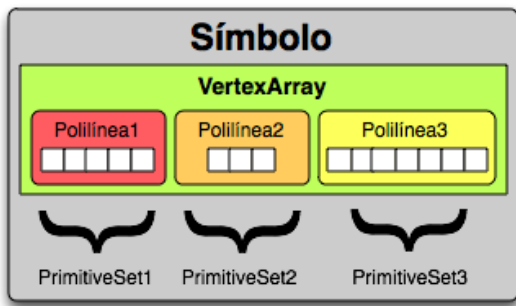
Figura 2: Estructura interna de un símbolo de tipo polilínea
