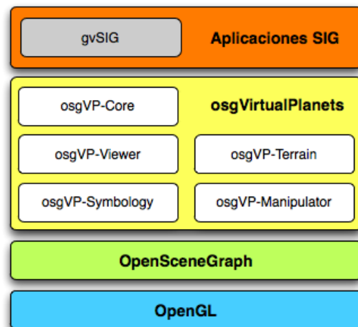
Figura 1: Arquitectura general de la librería osgVirtualPlanets
