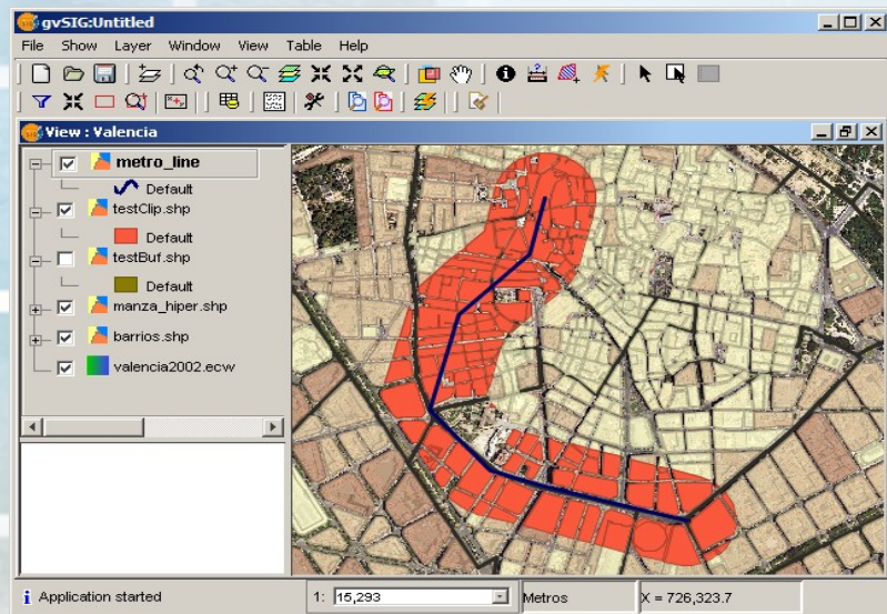
Desktop GIS
