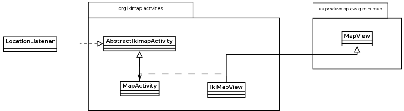
Fig 4. Ejemplo de implementación de clases en ikiMap para Android
