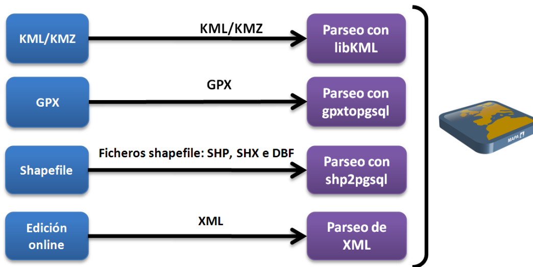
Figura 2: Mecanismos de introducción de datos geométricos
