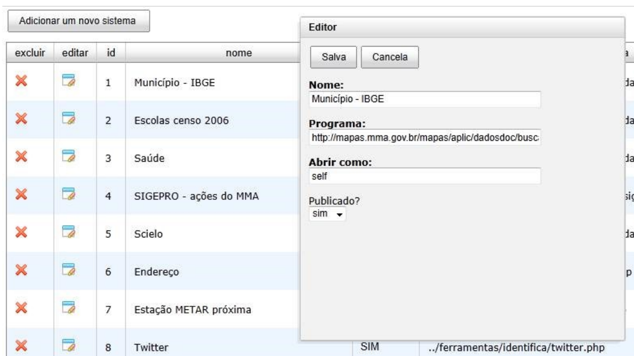
Ilustração 38: Editor de sistemas adicionais de identificação
