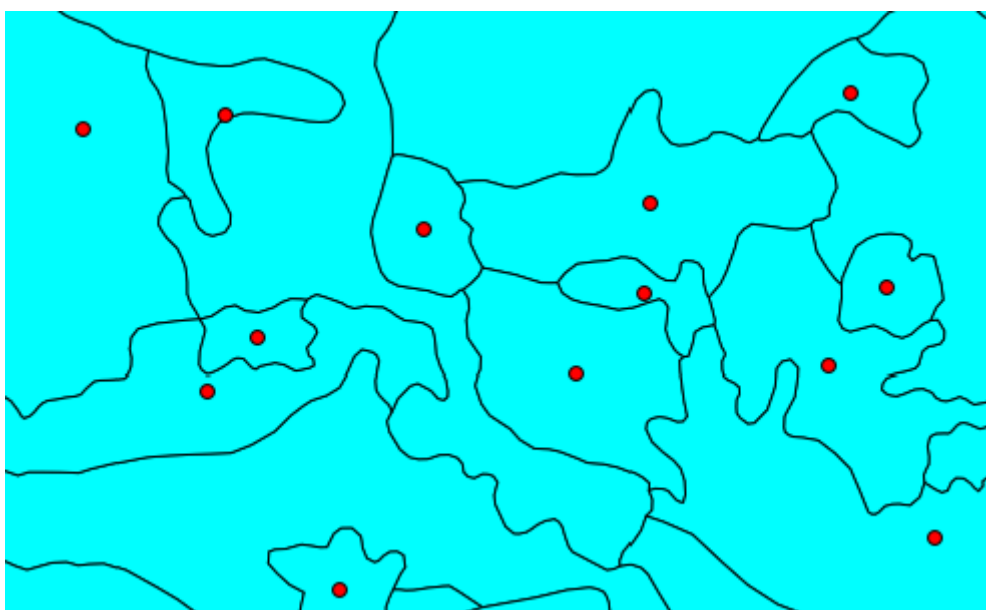
Ilustração 64: Centróides
