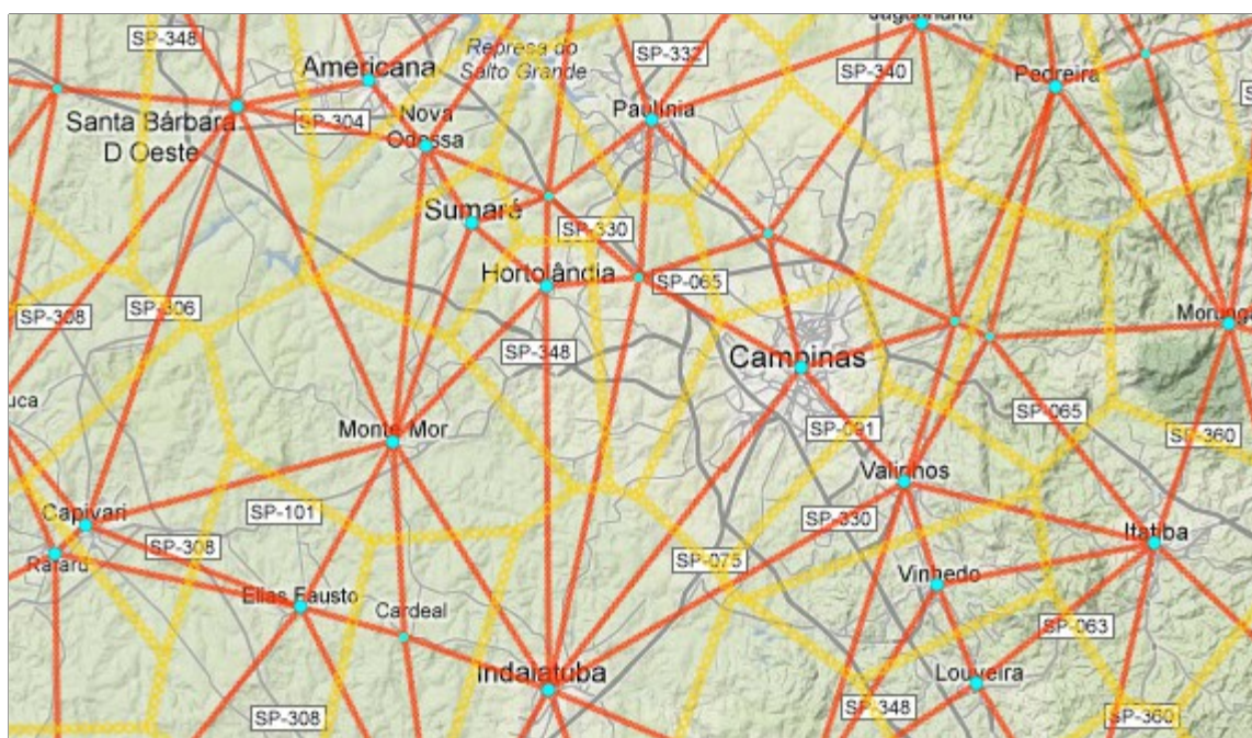
Ilustração 59: Triangulação
