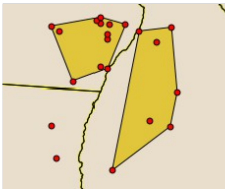
Ilustração 63: Agrupamento
