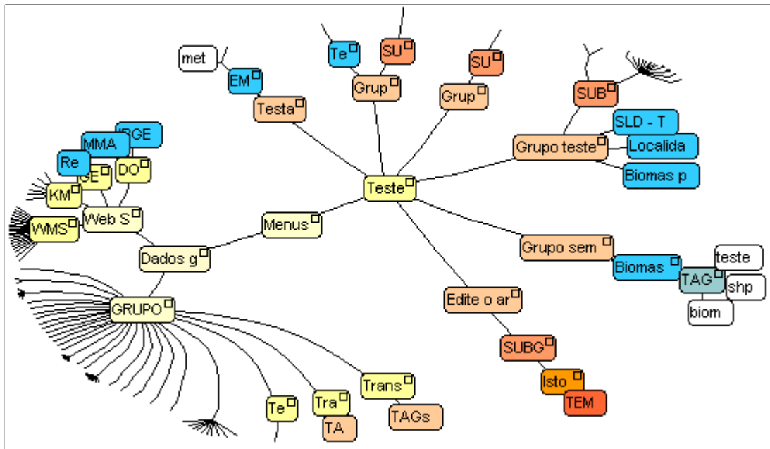
Ilustração 73: Árvore hiperbólica
