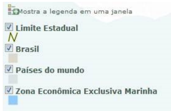
Ilustração 12: Guia "legenda"
