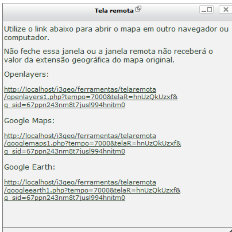
Ilustração 71: Tela remota
